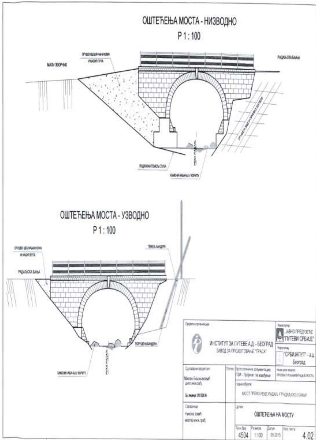
Оштећења на мосту
